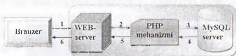
10.3-rasm. WEB ma'lumotlar bazasining bazali arxitekturasini o'zida WEB brauzer, WEB server, mexanizm sahifalari va ma'lumotlar bazasini jamlaydi.
