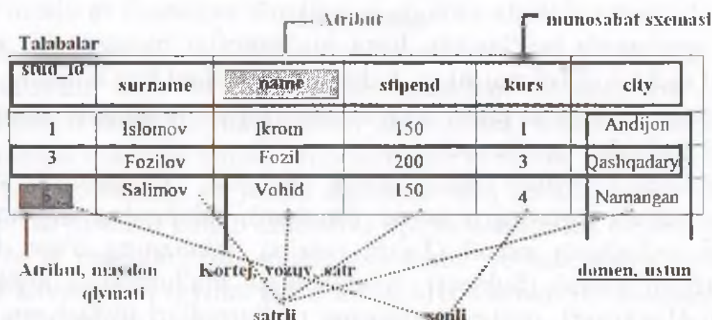
10.1-rasm. Jadval strukturasi
