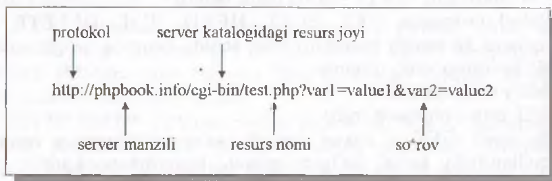
4.1-rasm. URLning to'liq shakli.
